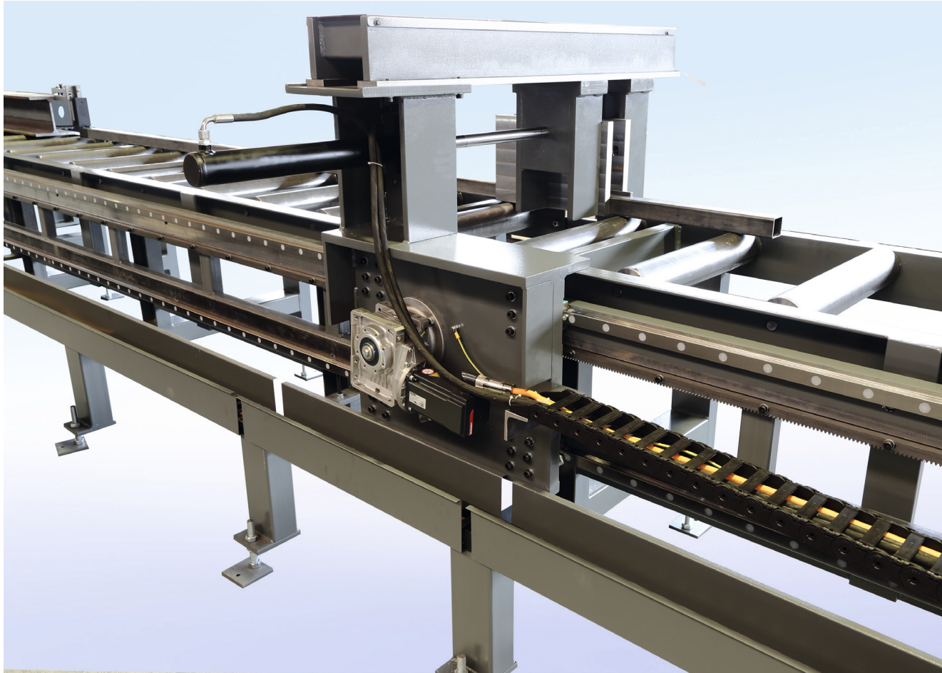
Materialvorschub durch Linearführung, Servomotor und Zahnstange
