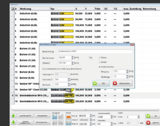
Eingabefeld der X und y Positionen mit Schnell-Werkzeugeingabe von Bohrer
