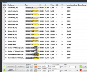
Eingabefeld der X und y Positionen mit Werkzeug
