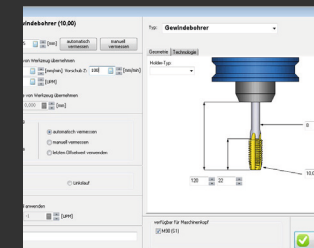
Maske der Werkzeugeingabe Fräser und Bohrer
