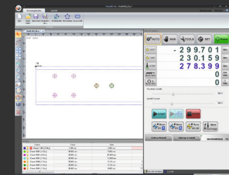
Bildschirm bei Startbeginn mit Anzeige der aktuellen Positionen
